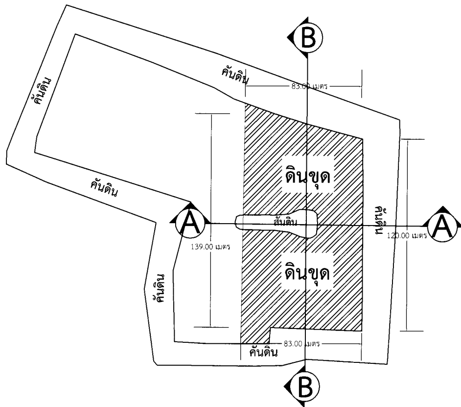
แปลนพื้นที่ (ขุดขยายและเพิ่มเติม)
